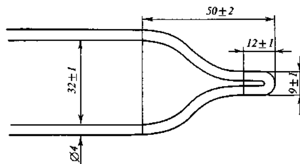
Fig. 1 Filament loop
