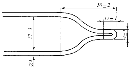
Fig. 1 Filament loop
