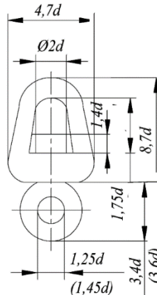
Fig. 7.1.3-7 Swivel
