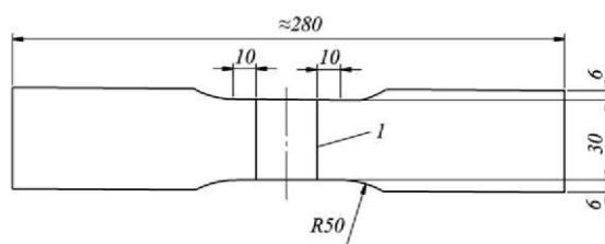
Fig. 4.2.8.5-2 Tensile test specimen: 1 — weld edge
